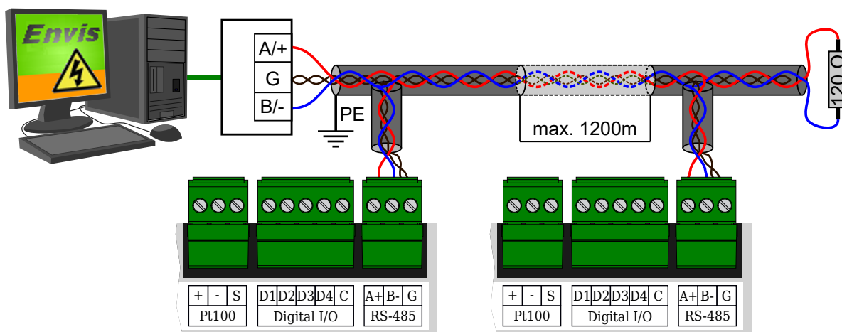
Obrázek 7: Zapojení komunikačních linek sběrnice RS-485 přístrojů ARTIQ 233.
